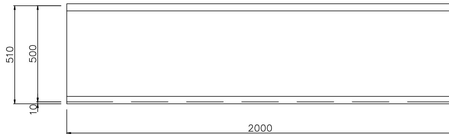
全景図 (S=1/6)
