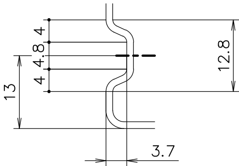
リブ詳細 (S=3/1)
