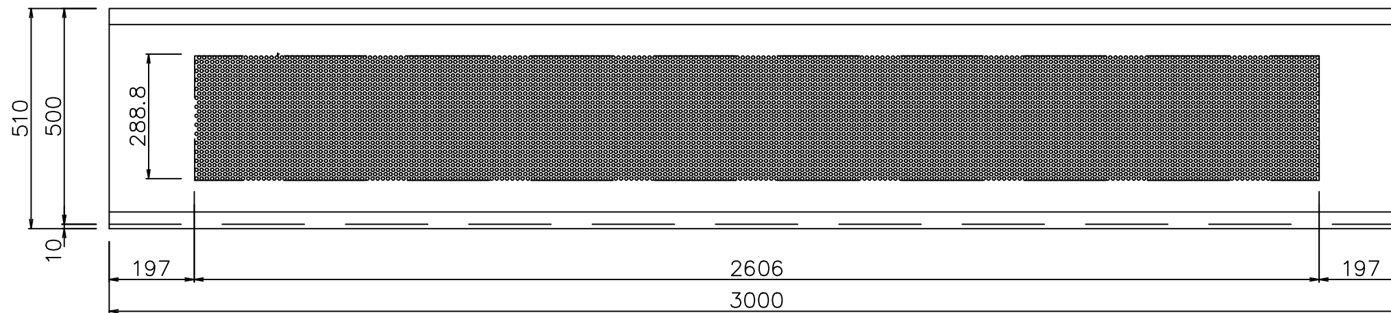
全景図 (S=1/6)
