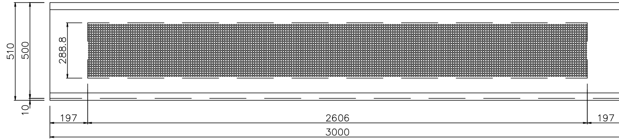
全景図 (S=1/6)
