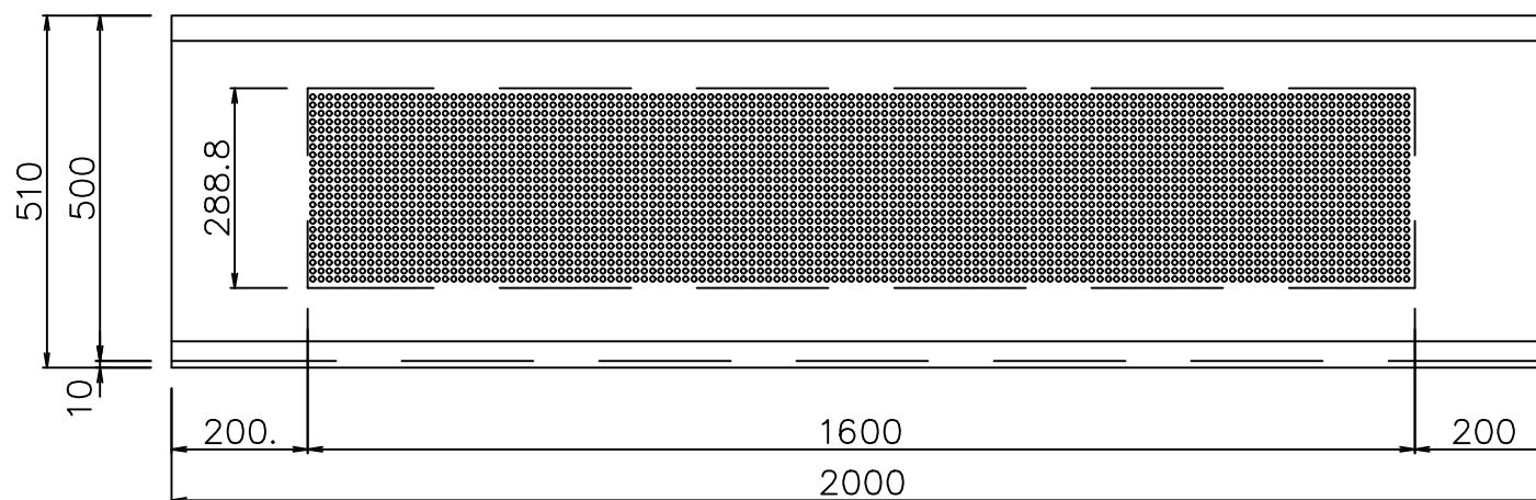
全景図 (S=1/6)
