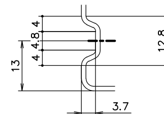
リブ詳細(S=3/1)
