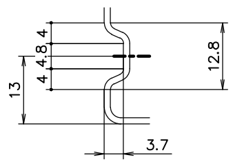
リブ詳細(S=3/1)
