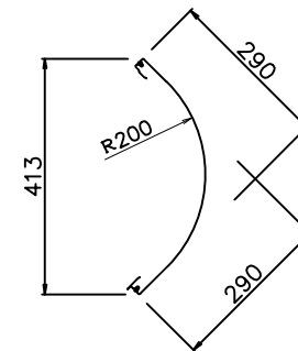
リブ詳細(S=3/1)
