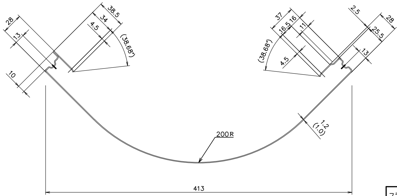
断面詳細図 (S=1/1)
