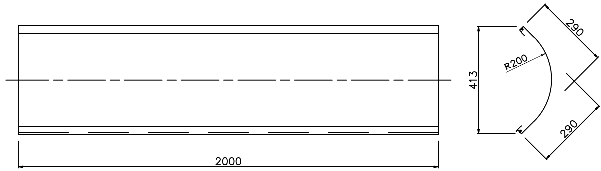
全景図 (S=1/6)
