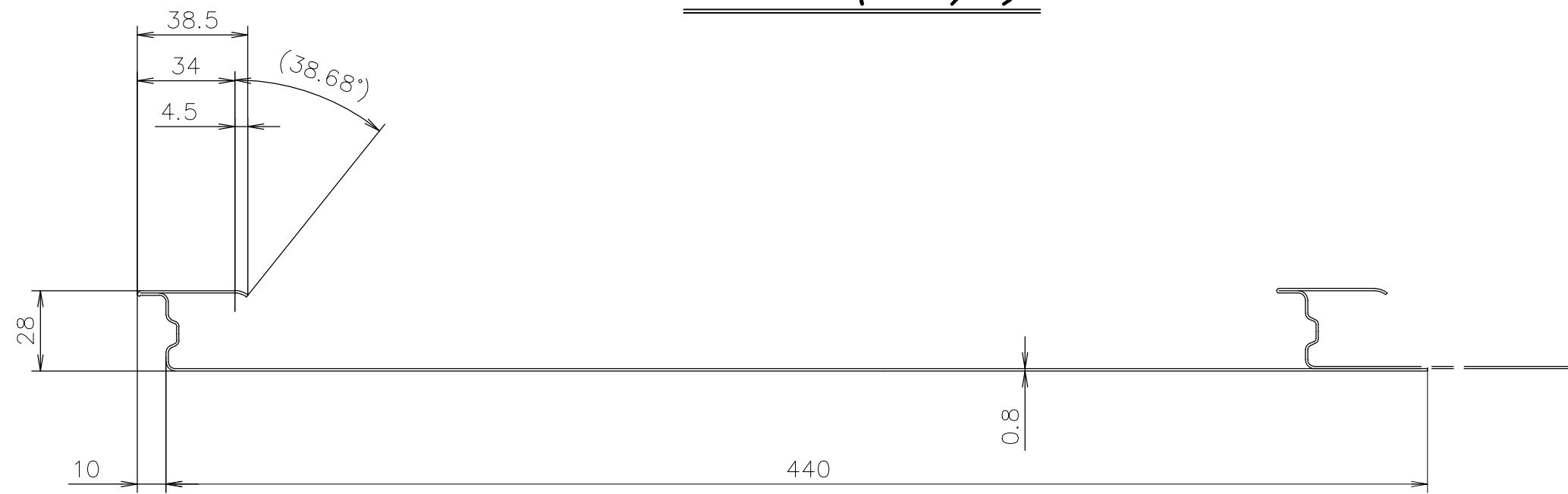
断面詳細図 (S=1/1)
